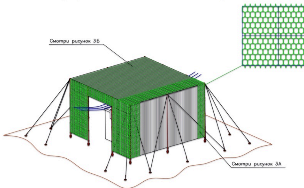
СХЕМА 4 ЭТАП № 4: СПЛОШНАЯ УКЛАДКА СЕТКИ МАНТЬЕ 100×80 ММ С ДВУОСНЫМ ТРОСОВЫМ УСИЛЕНИЕМ И ФИКСАЦИЕЙ
