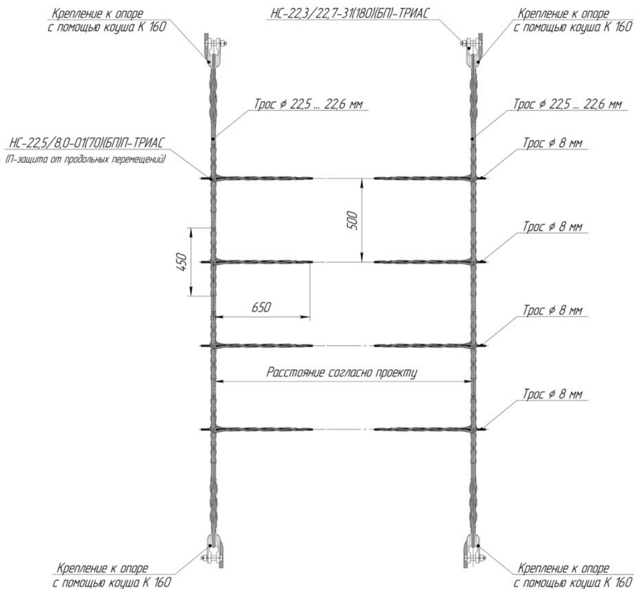
РИС. 1А КРЕПЛЕНИЕ СИЛОВЫХ ТРОСОВ Ø 22,5...22,6 мм И СЕТКИ ТРОСОВ Ø 8 мм (ВЕРХНЯЯ ЧАСТЬ ЗАЩИТЫ)
